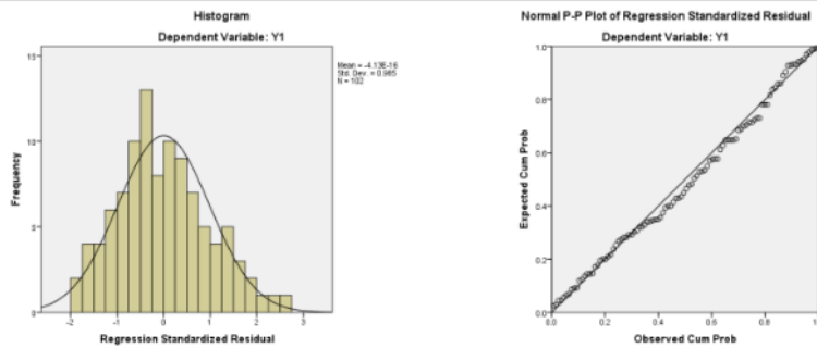
Gambar 1 Histogram dan Normal P-P Plot
